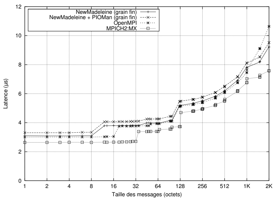
FIGURE 7.7 – Impact de PIOMAN sur la latence du réseau MYRINET
